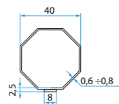
A3505_0501 Adapteri za osmerokutne cijevi 40 (vanjska kopča)
