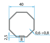
A3505_0502 Adapteri za osmerokutne cijevi 40 (unutarnja kopča)
