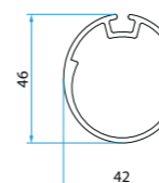
A3505_0508 Adapteri za ovalne cijevi 42x46
