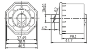
A3515_5179 Osmerokutna remenica 40 u stanju mirovanja
